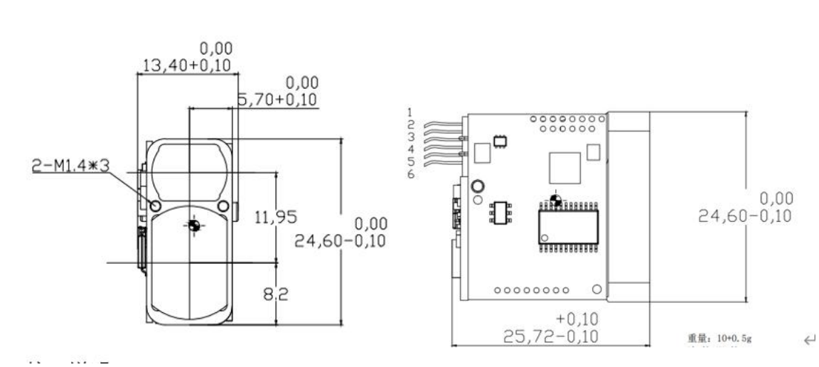
图 4-1 模块引脚
