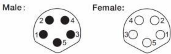
图 4 接口示意
