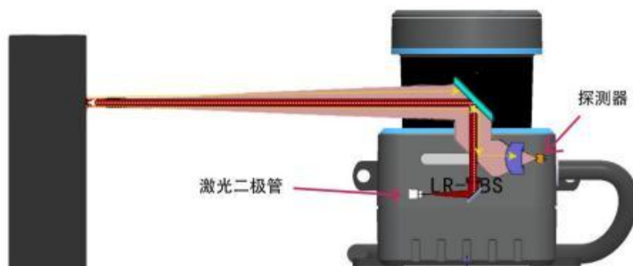
图 9 LR-1BS5 激光雷达工作示意图
