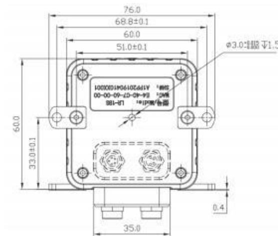
图 2 LR-1BS5 底部安装接口
