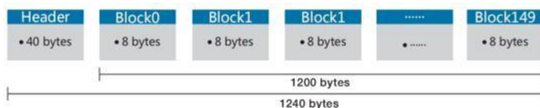
图 1 点云信息数据包格式
